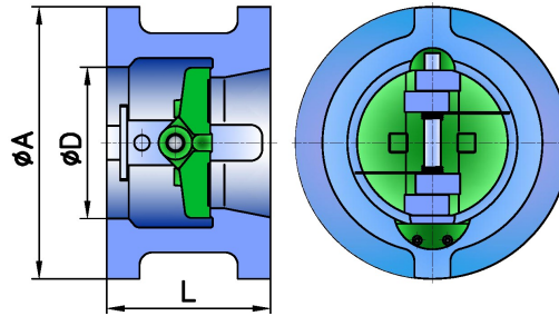
ТИП „WAFER“
