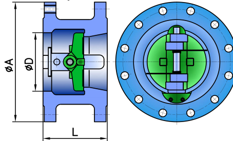
ФЛАНЦЕВОЕ ИСПОЛНЕНИЕ
